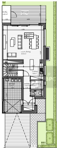
REZ-DE-CHAUSSEE E 1:100
