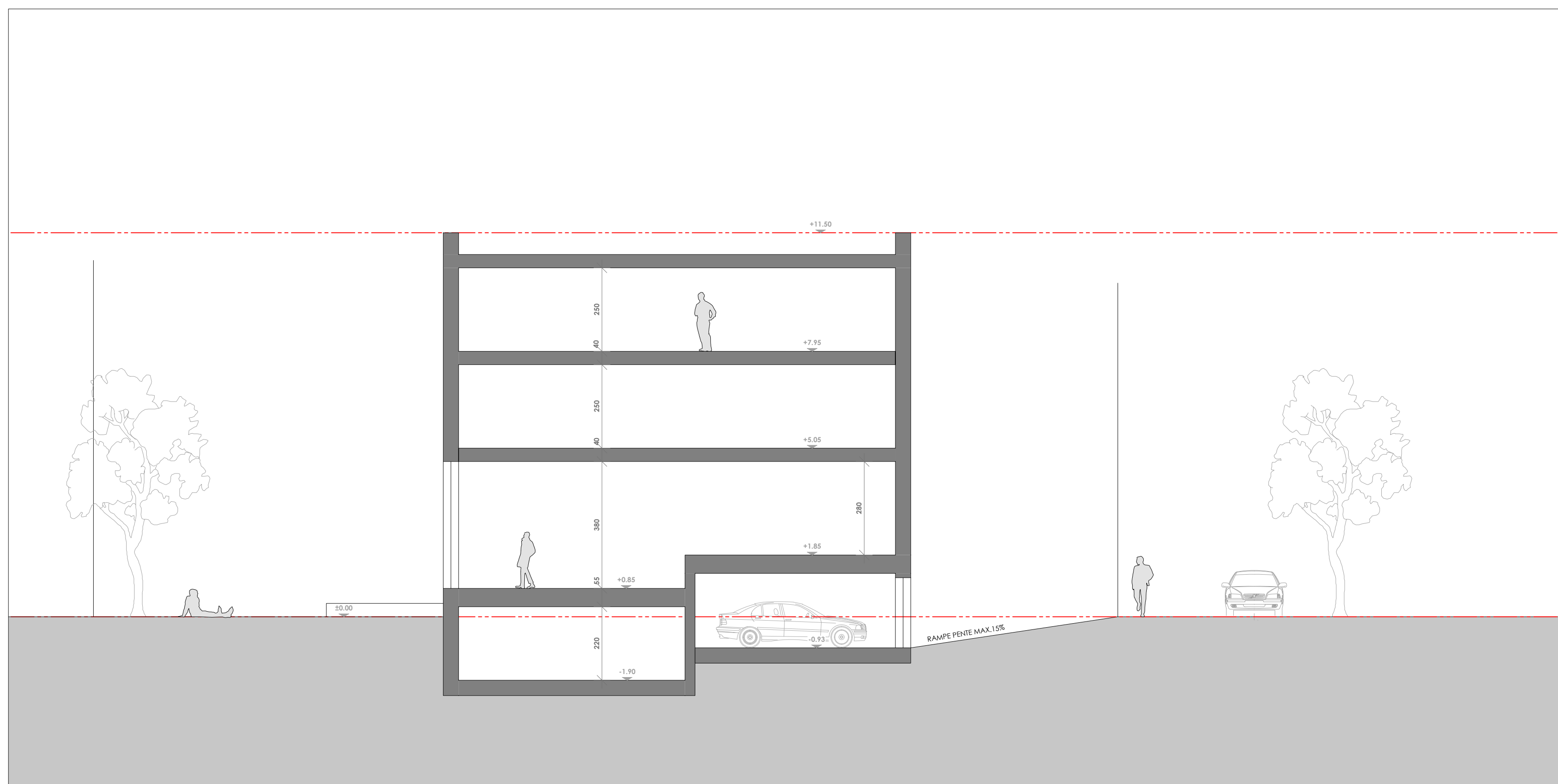
COUPE A-A
