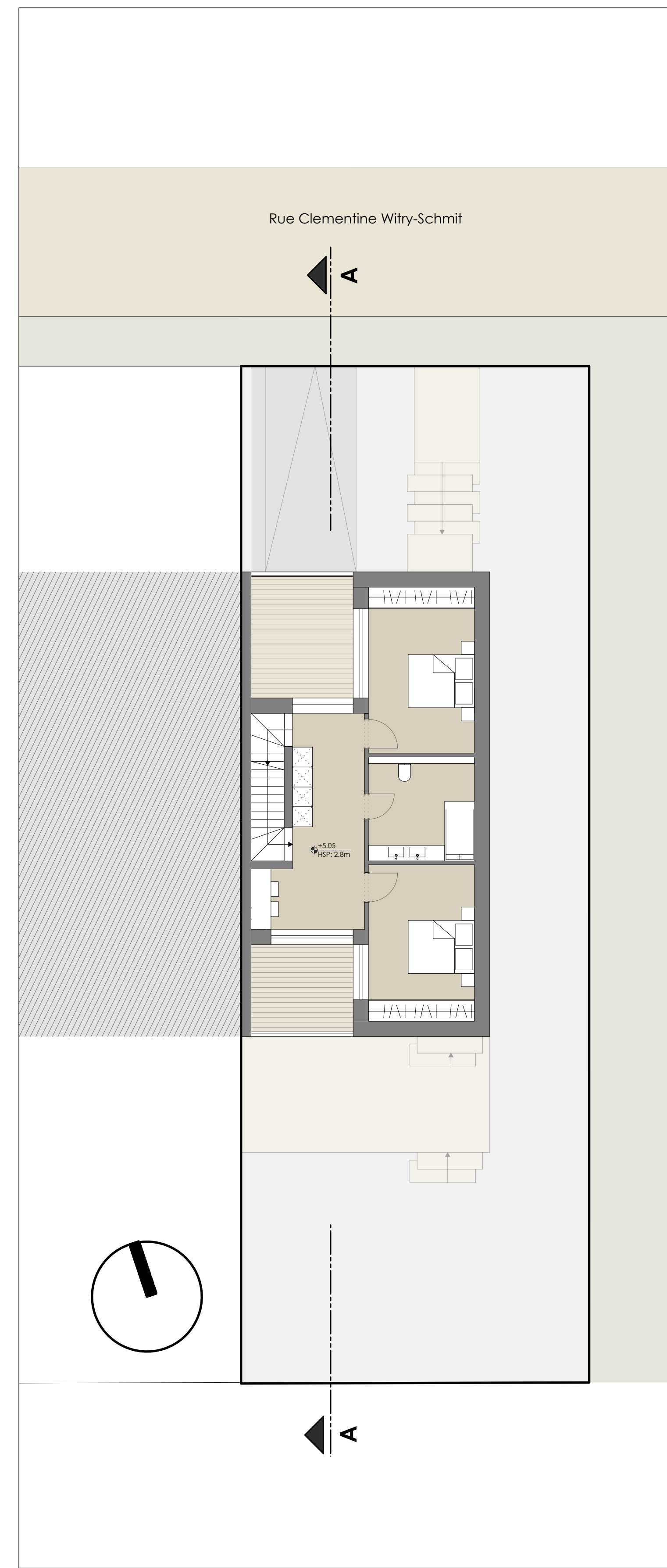
ETAGE 1
