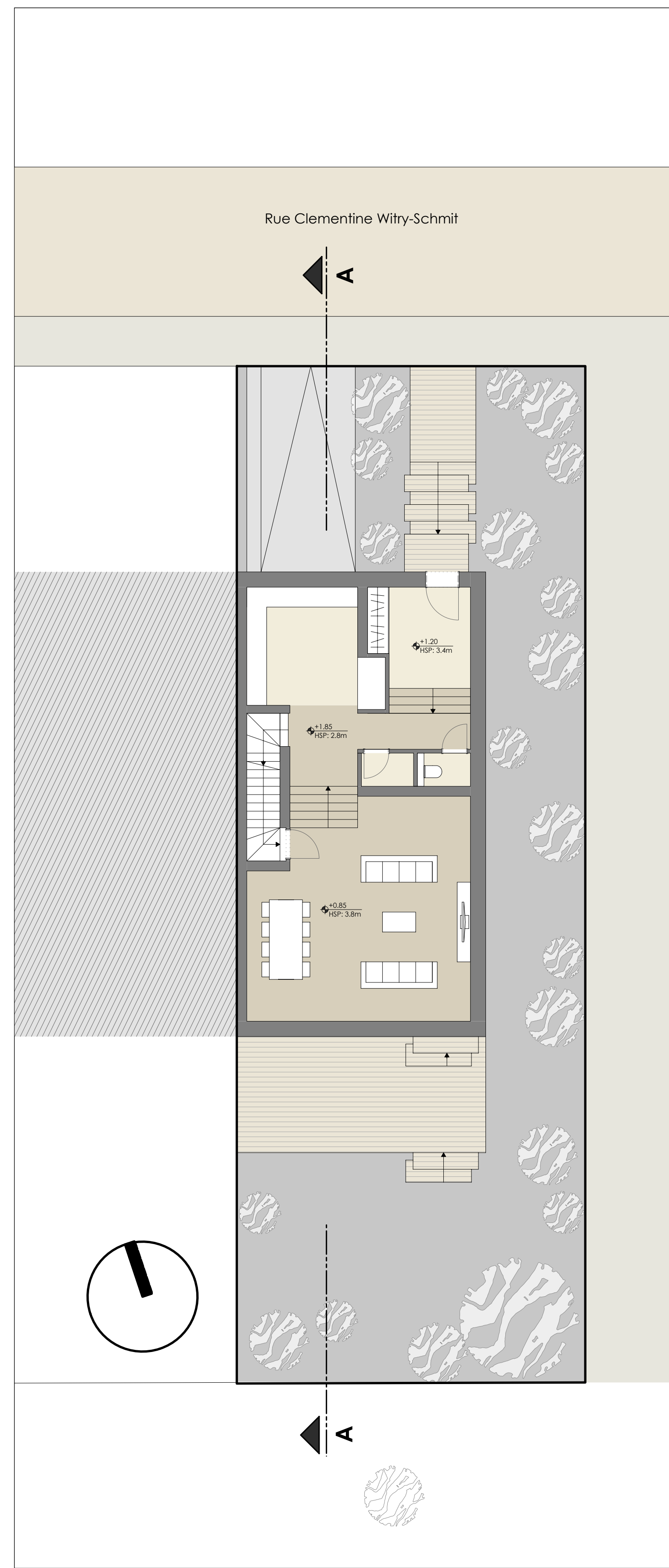
REZ-DE-CHAUSSEE
